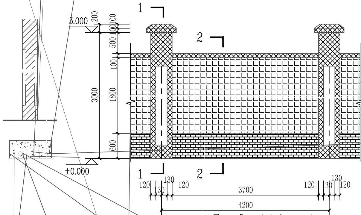
3-6 段围墙立面图
